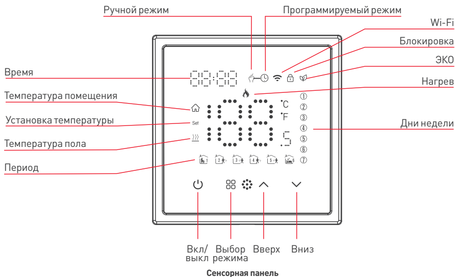
Рис. 4. Назначение индикаторов и кнопок на сенсорной панели
