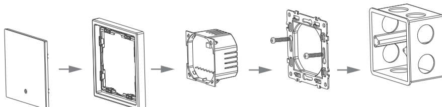
Рис. 2. Монтаж терморегулятора
