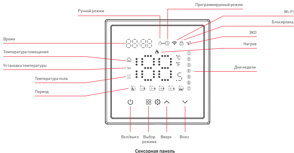
Рис. 4. Назначение индикаторов и кнопок на сенсорной панели
