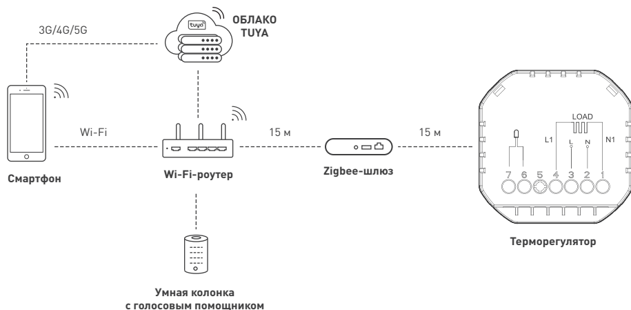
Рис. 1. Структурная схема построения системы
