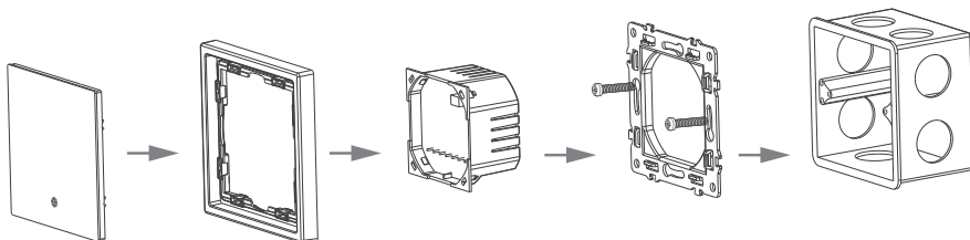
Рис. 2. Монтаж терморегулятора
