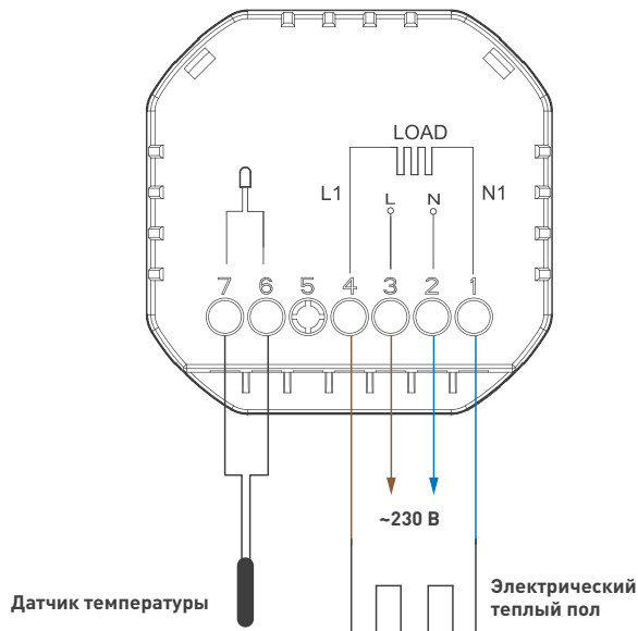
Рис. 3. Схема подключения терморегулятора
