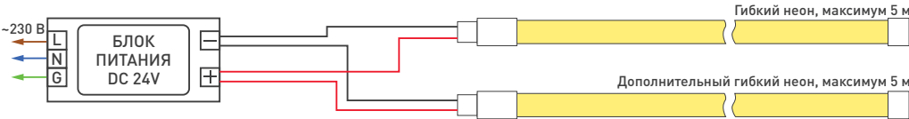
Схема 1. Подключение гибкого неона
