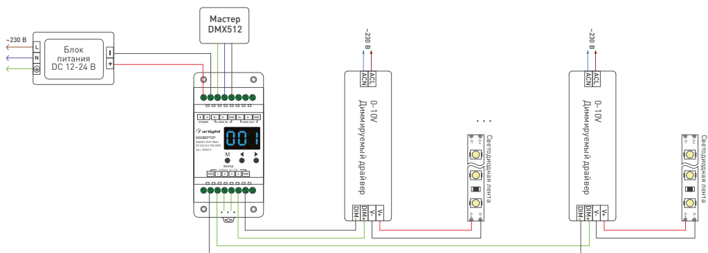
Рисунок 1. Схема подключения конвертера SMART-K39-DMX
