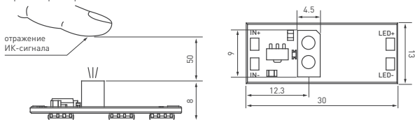
Рис. 1. Чертеж и габаритные размеры.
